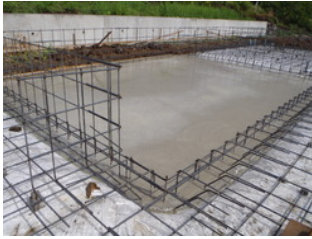
①土間コンクリート
