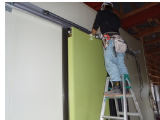
⑳大扉調整据付
