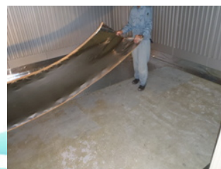
⑫防湿RAシート
